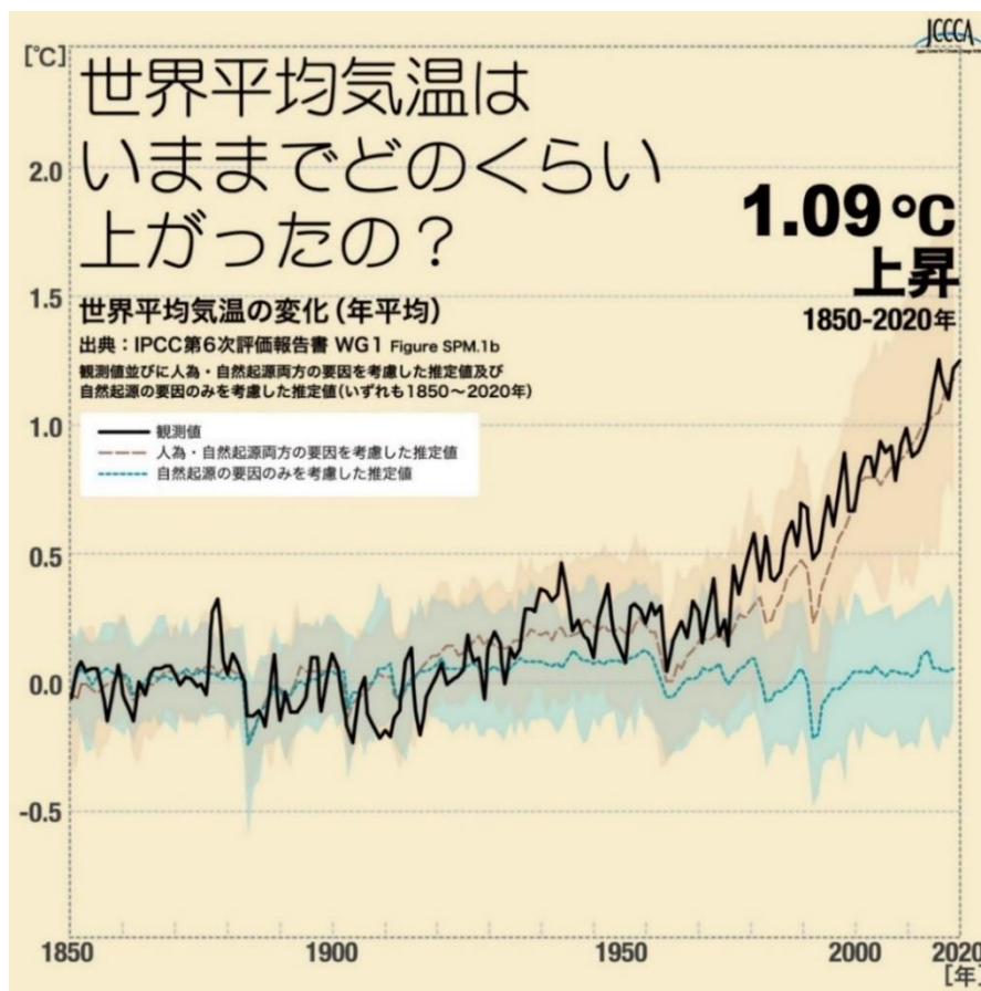
図 1-2 世界平均気温の変化（1850～2020 年・観測） 出典：全国地球温暖化防止活動推進センター
