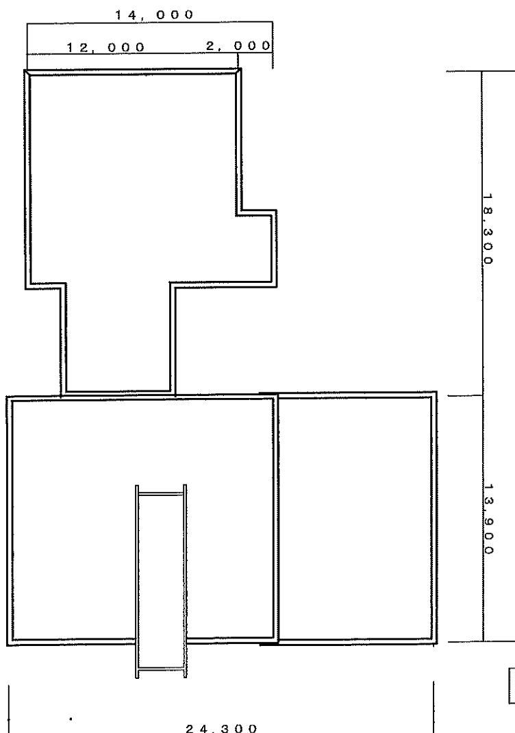
平面図
