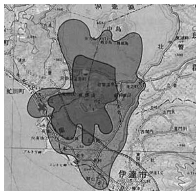
1822 年の有珠山噴火で発生した火砕流の範囲 ※ここでは火砕サージも含めて「火砕流」と表現しています。
