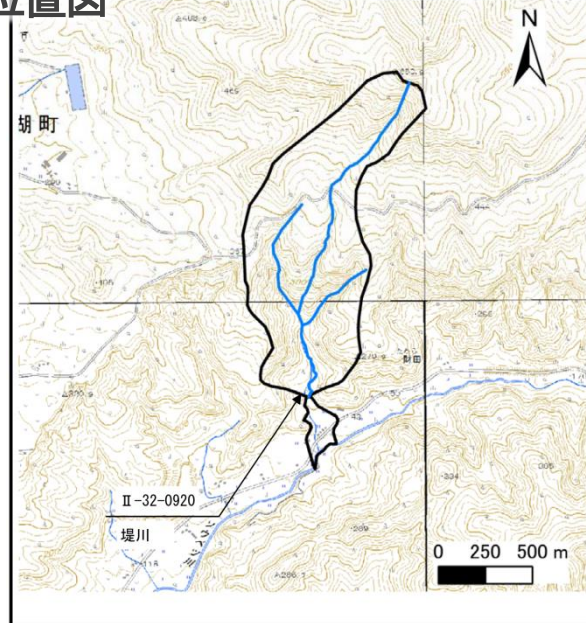
位置図 (1/25,000)
