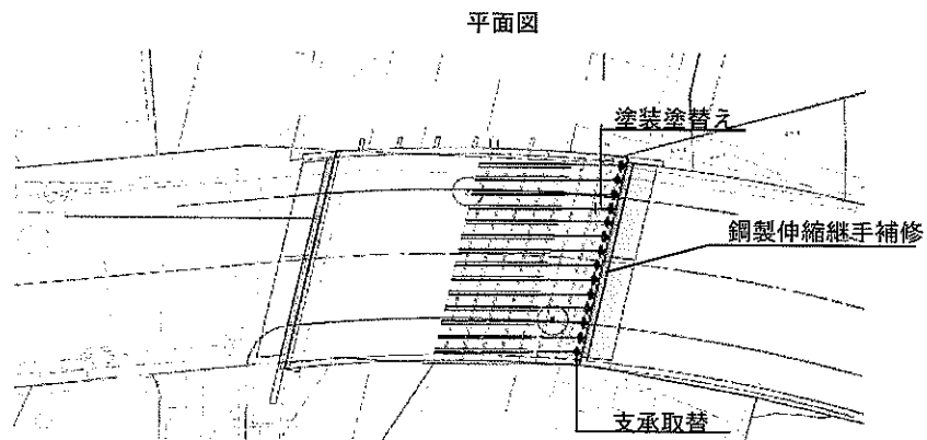
橋梁補修一般図
